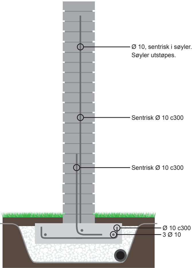
Fig. 3: Rette murer og murer med ensidig belastning bør ha et armert fundament som Tenso Multimur-elementene forankres i. Størrelse på fundamentet avhenger av vegghøyden. Sålen må være minimum 20 cm tykk og 60 cm bred. Maksimum høyde på muren er 2,2 meter.
