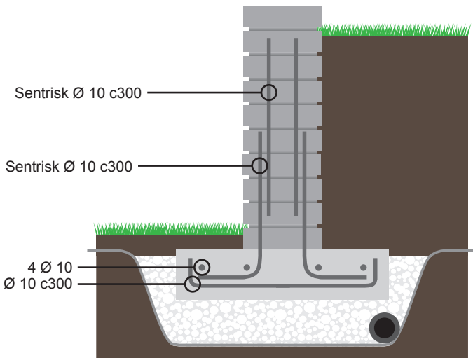
Fig. 2: Når Tenso Multimur brukes som støttemur må den ha dobbelarmering slik som vist på illustrasjonen over. Størrelse på fundamentet avhenger av vegghøyden. Sålen må være minimum 20 cm tykk og 60 cm bred. Drenerende masse legges inntil muren.
