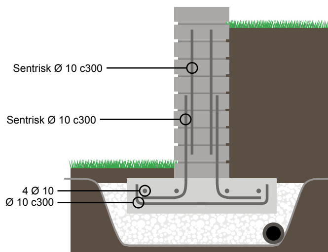
Fig. 2: Når Tenso Multimur brukes som støttemur må den ha dobbelarmring slik som vist på illustrasjonen over. Størrelse på fundamentet avhenger av veggghøyden. Sålen må være minimum 20 cm tykk og 60 cm bred. Drenerende masse legges inntil muren.
